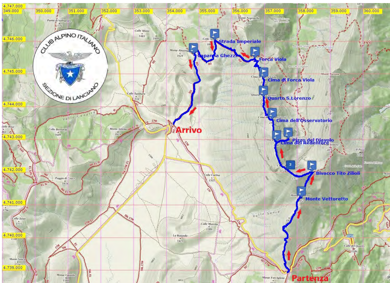
Traversata da Forca di Presta a Castelluccio (x => km, y => m)
